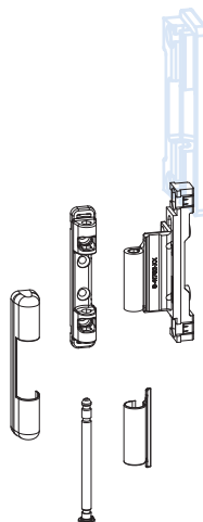
Опора верхняя + ось Петля средняя Накладки: опоры верхней 9-41653-00-0- петли средней 9-41695-00-0-*
