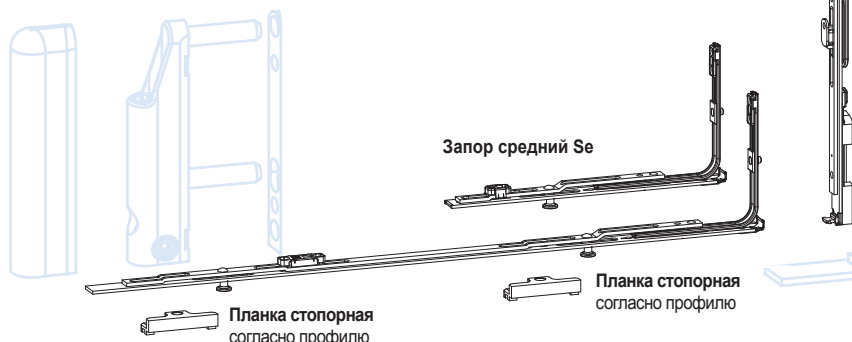
Передача фальцевая рычажная ZH-GK
